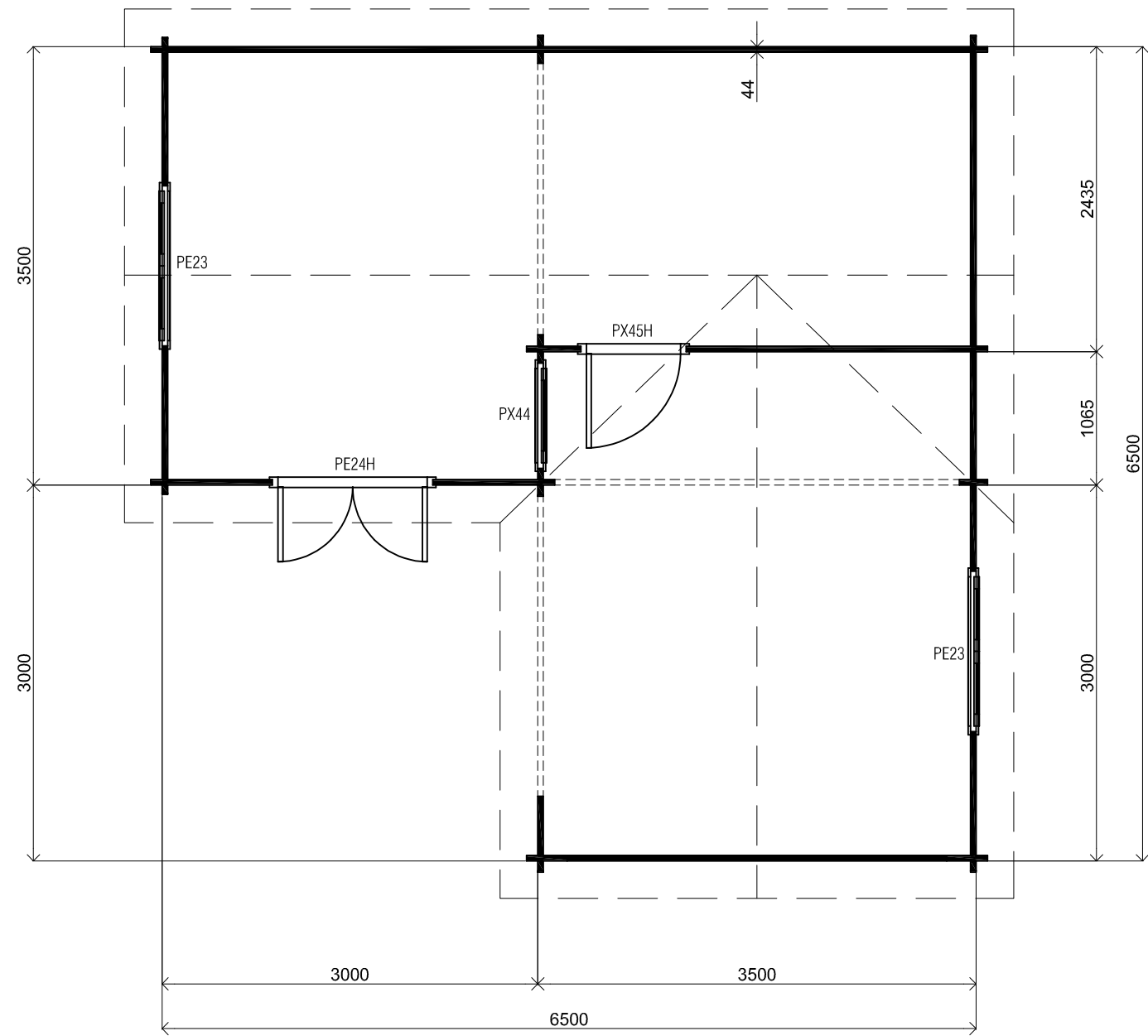
Plattegrond / Plan
