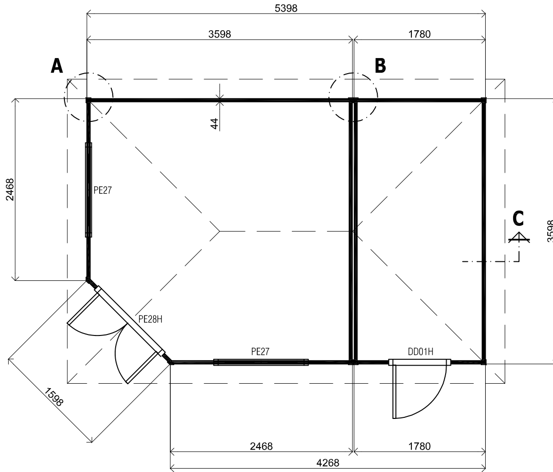
Plattegrond / Plan
