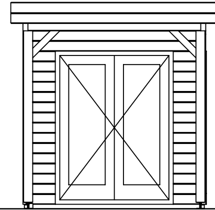
(L) Zijaanzicht / Side view / Seiten ansicht
