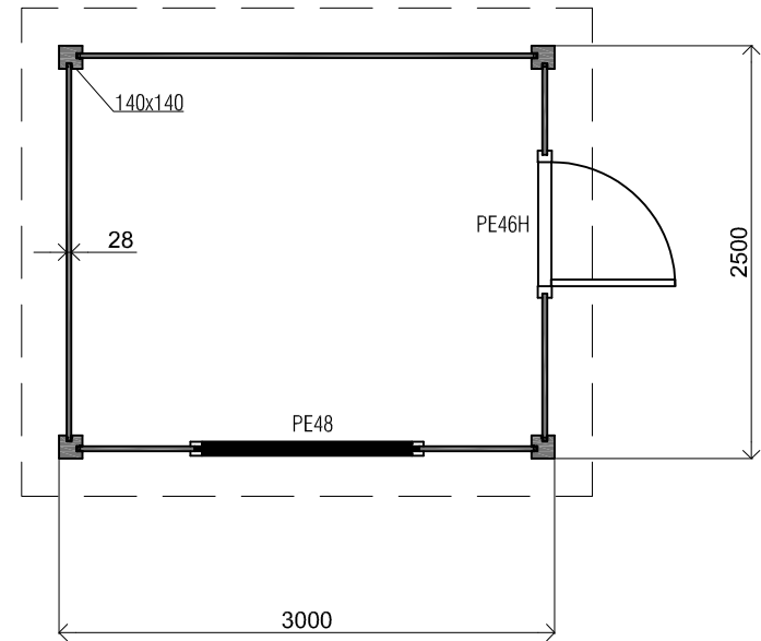
Plattegrond / Plan
