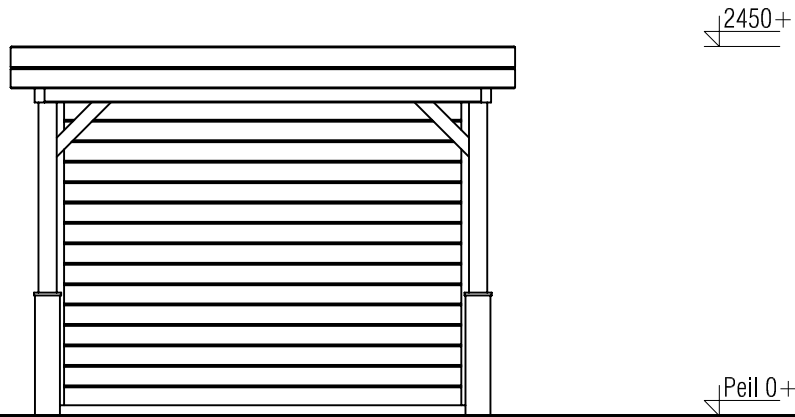
Voorraanzicht / Front view / Vorderansicht
