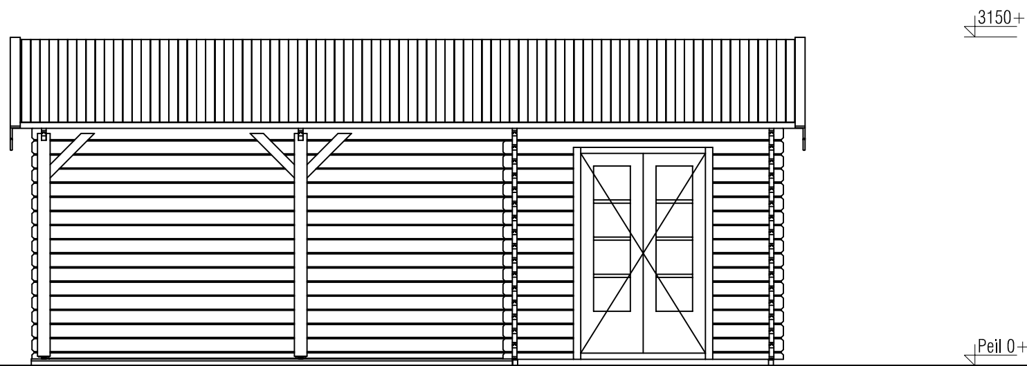
Vooraanzicht / Front view / Vorderansicht
