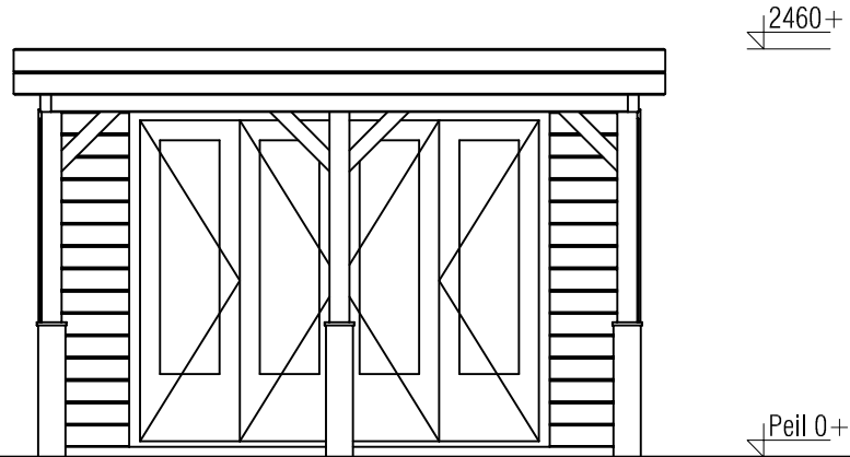
Voorbeeld / Front view / Vorderansicht
