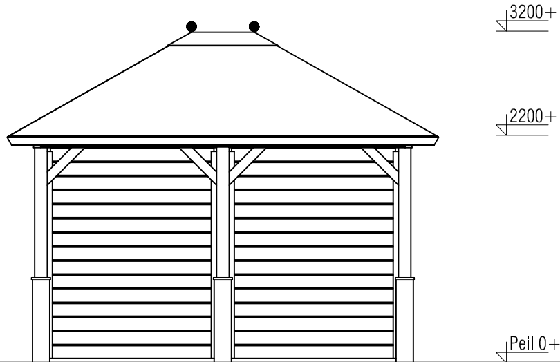
Voorzicht / Front view / Vorderansicht
