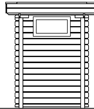
(R) Zijaanzicht / Side view / Seiten ansicht
