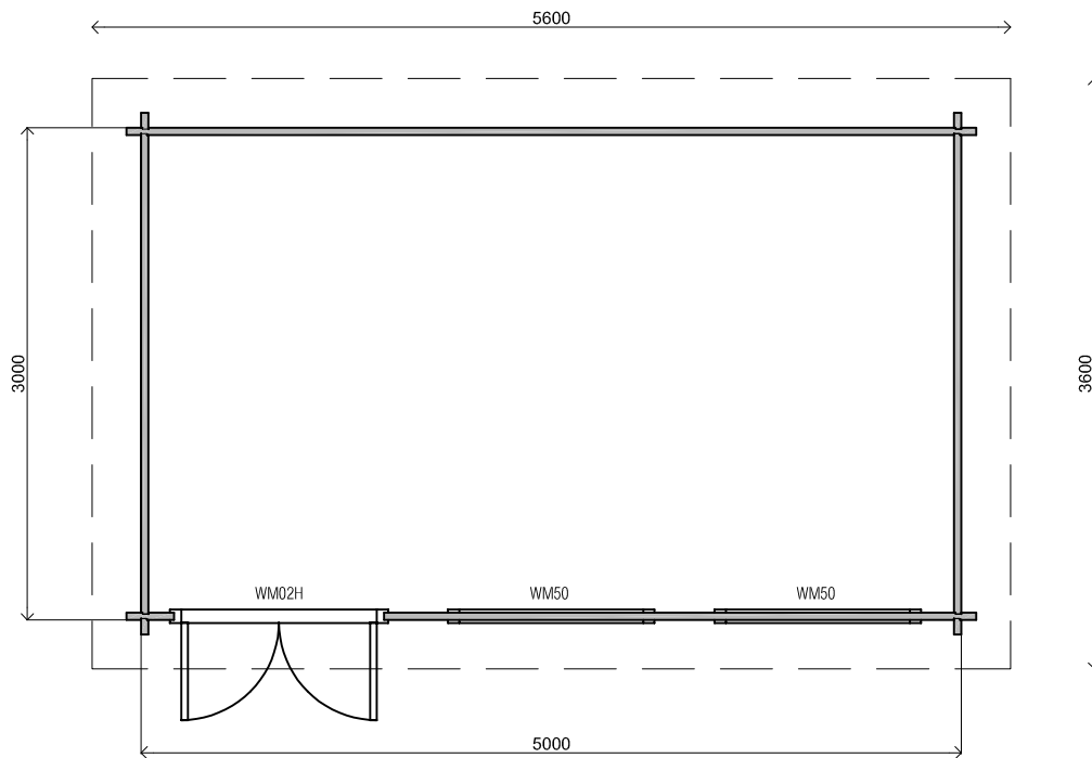
Plattegrond / Plan
