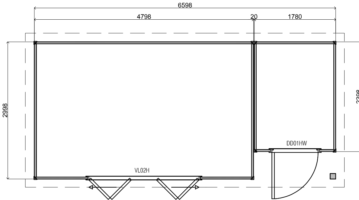
Plattegrond / Plan
