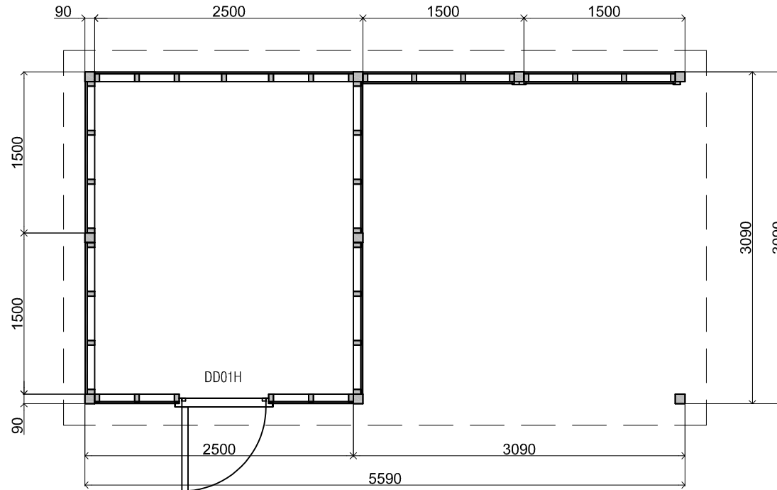
Plattegrond / Plan
