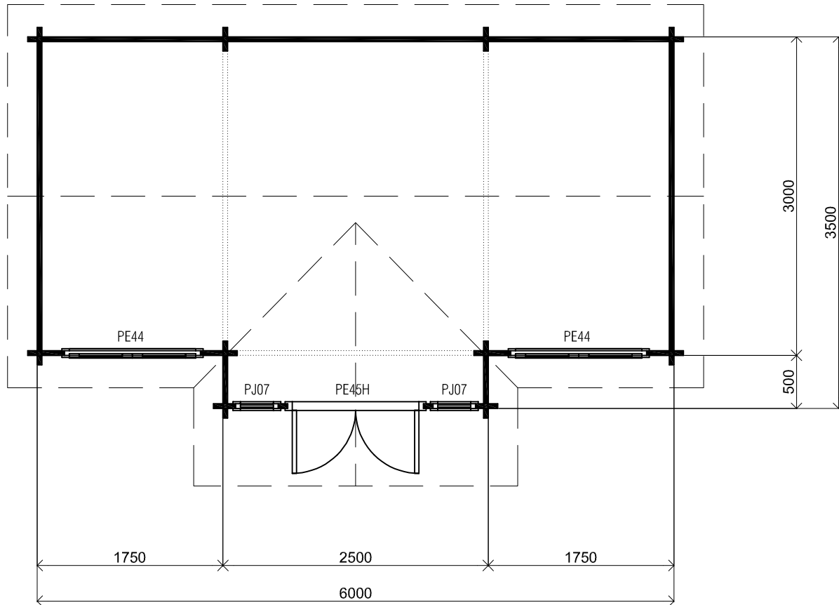
Plattegrond / Plan
