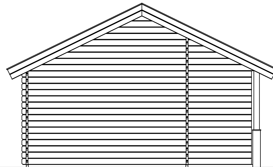
(L) Zijaanzicht / Side view / Seiten ansicht
