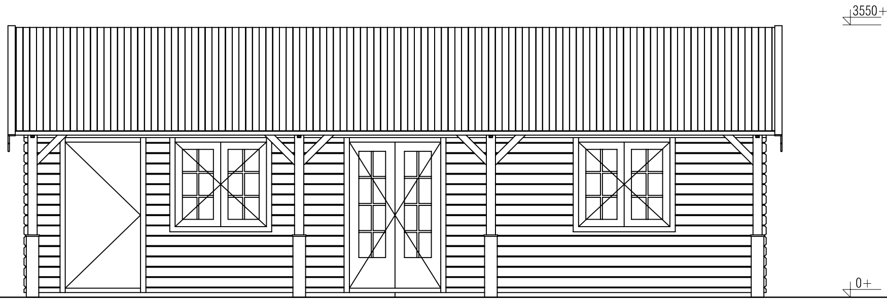
Voorraanzicht / Front view / Vorderansicht
