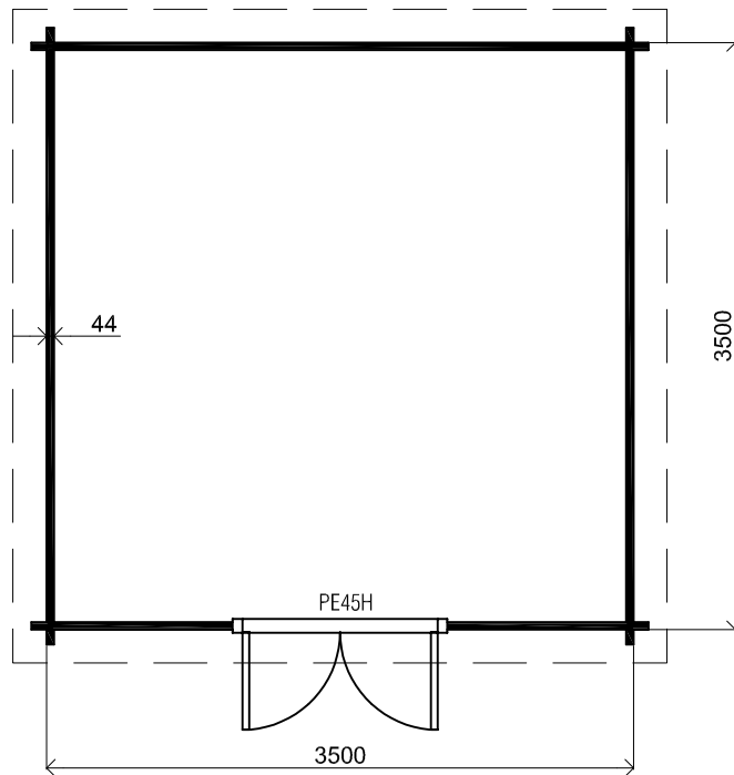
Plattegrond / Plan
