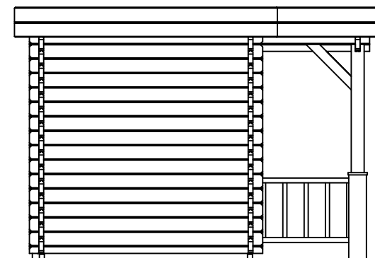
(L) Zijaanzicht / Side view / Seiten ansicht
