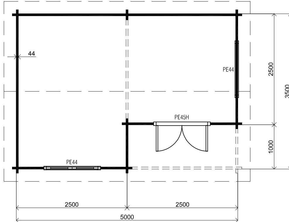
Plattegrond / Plan
