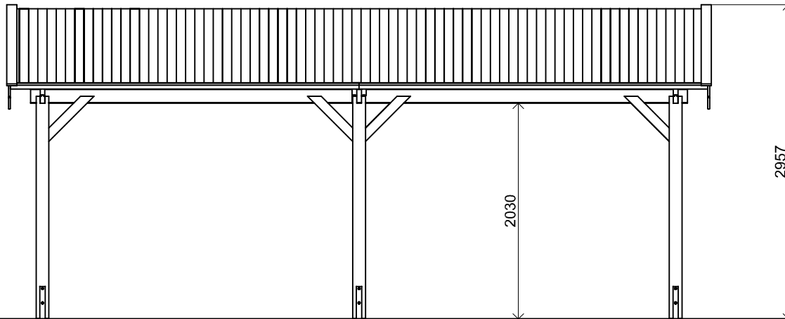
Zijaanzicht / Side view / Seiten ansicht
