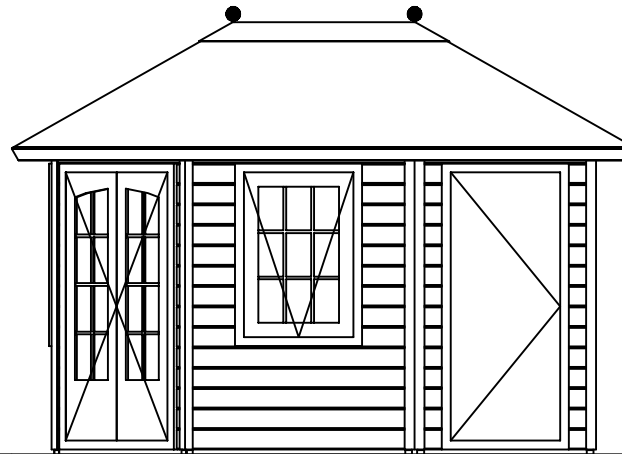
Vooraanzicht / Front view / Vorderansicht
