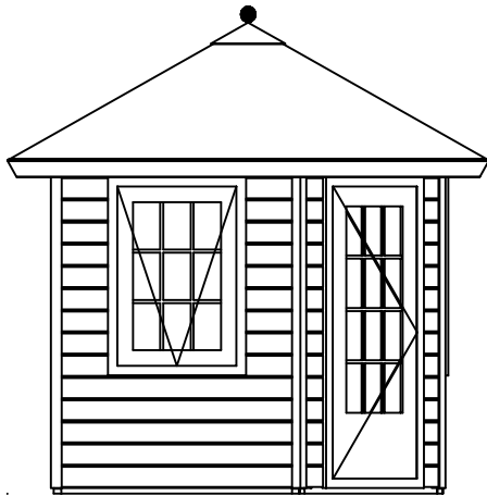
(L) Zijaanzicht / Side view / Seiten ansicht
