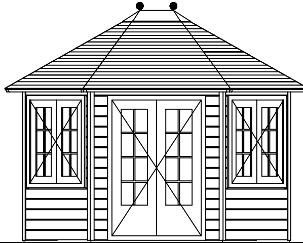
Vooraanzicht / Front view / Vorderansicht
