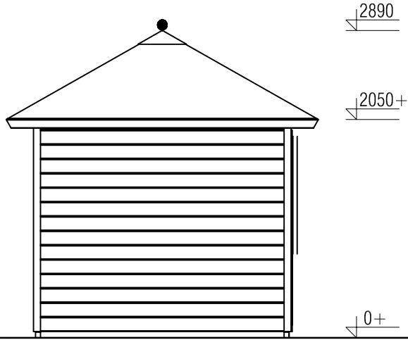
(L) Zijaanzicht / Side view / Seiten ansicht
