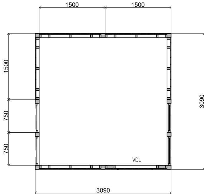
Plattegrond / Plan
