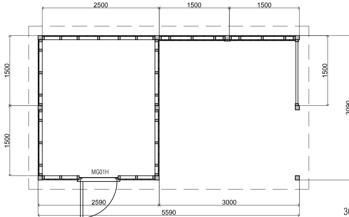
Plattegrond / Plan
