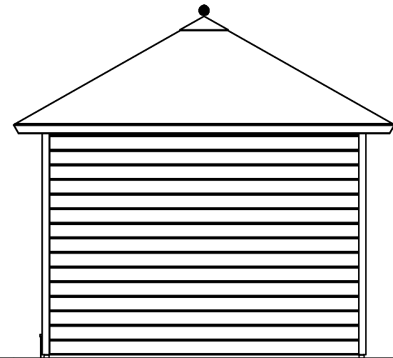
(R) Zijaaanzicht / Side view / Seiten ansicht
