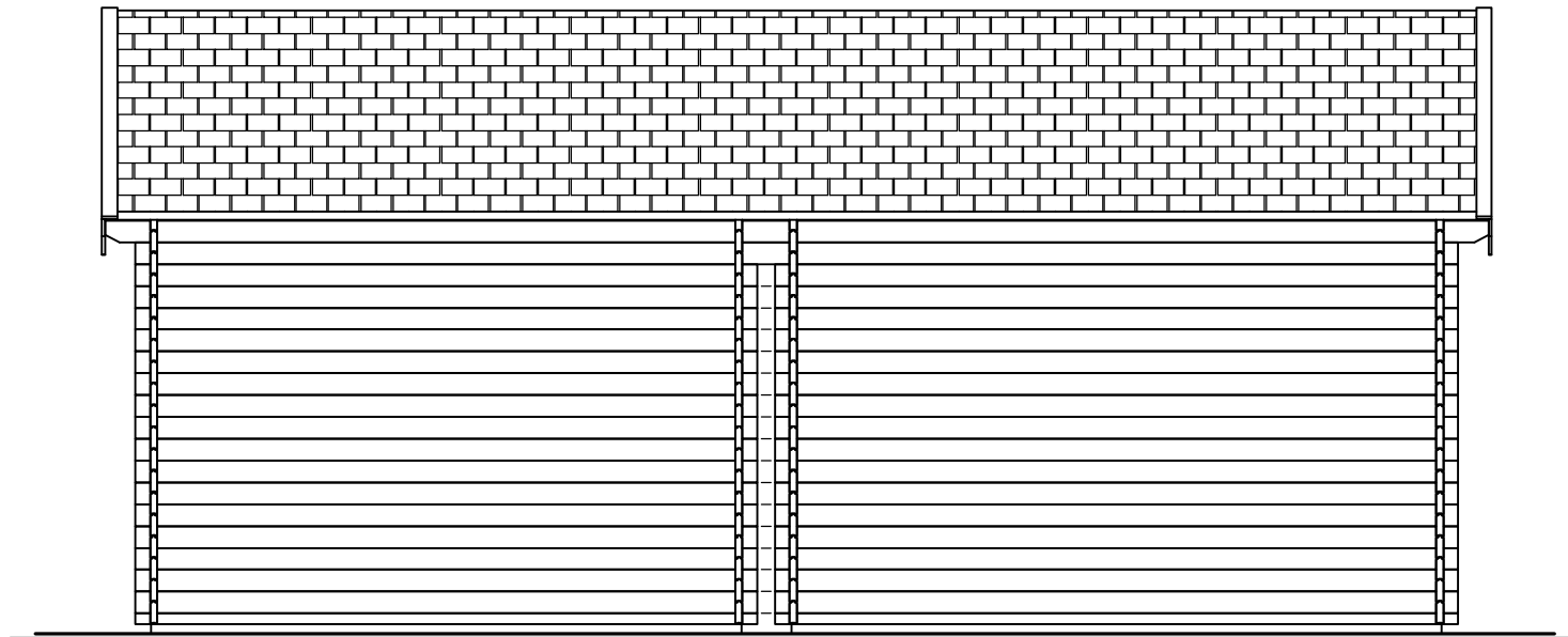
zij aanzicht (I) side view (I)
