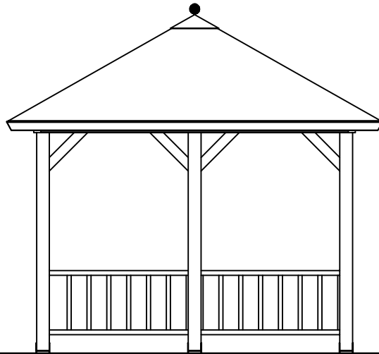
Vooraanzicht / Front view / Vorderansicht
