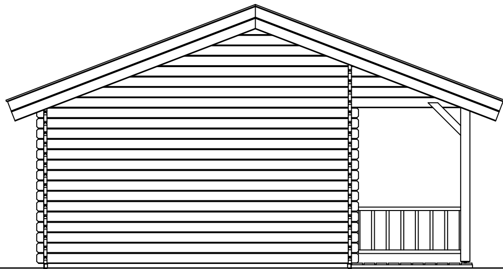
(L) Zijaanzicht / Side view / Seiten ansicht
