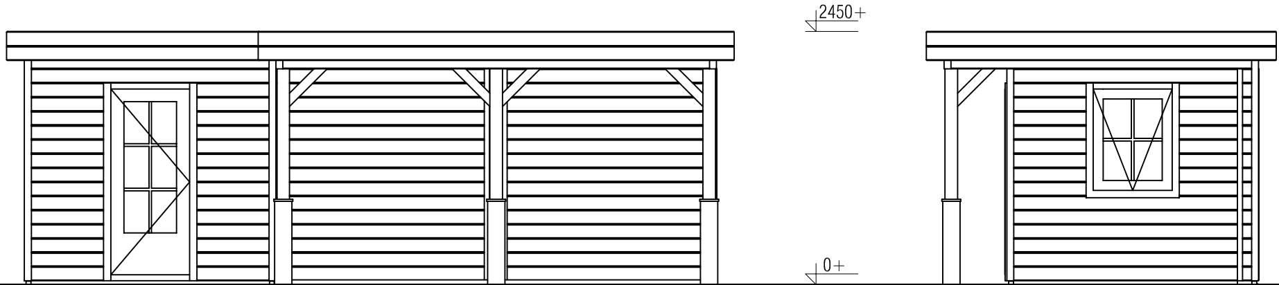
Vooraanzicht / Front view / Vorderansicht
