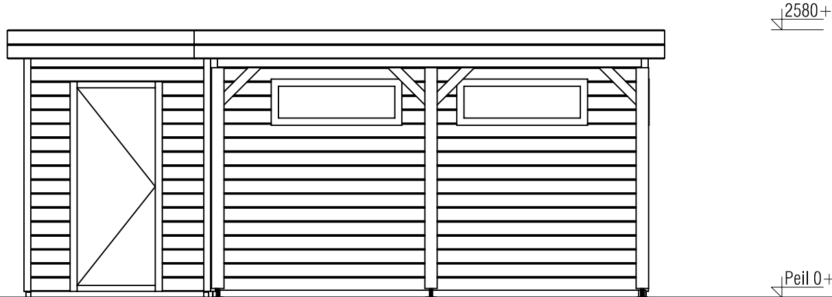
Vooraanzicht / Front view / Vorderansicht
