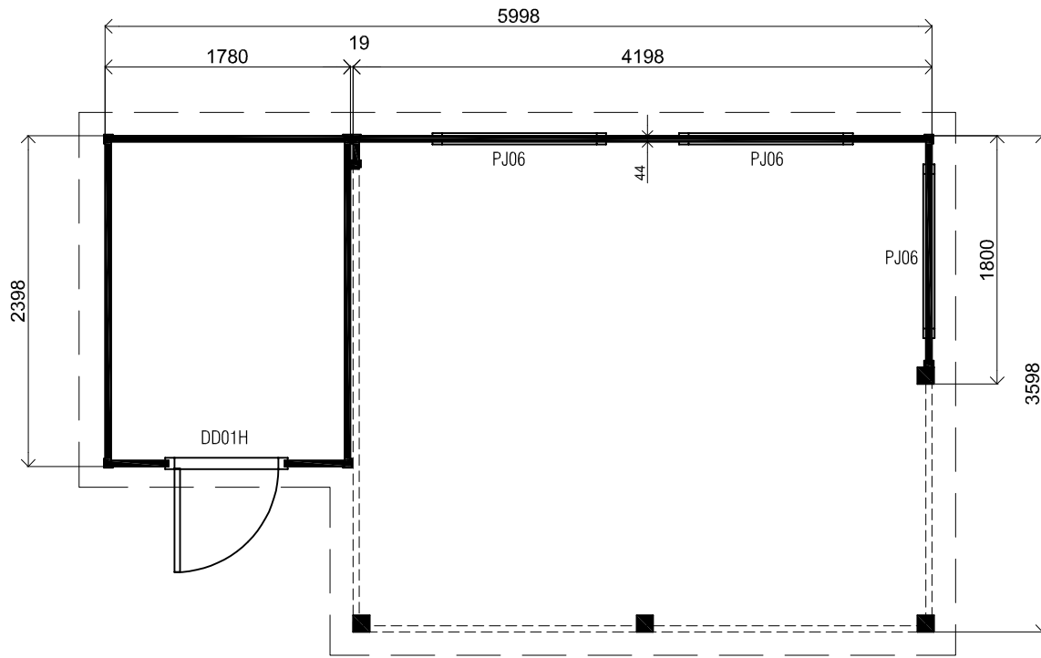
Plattegrond / Plan
